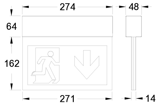
Maßzeichnung (Angaben in mm)
