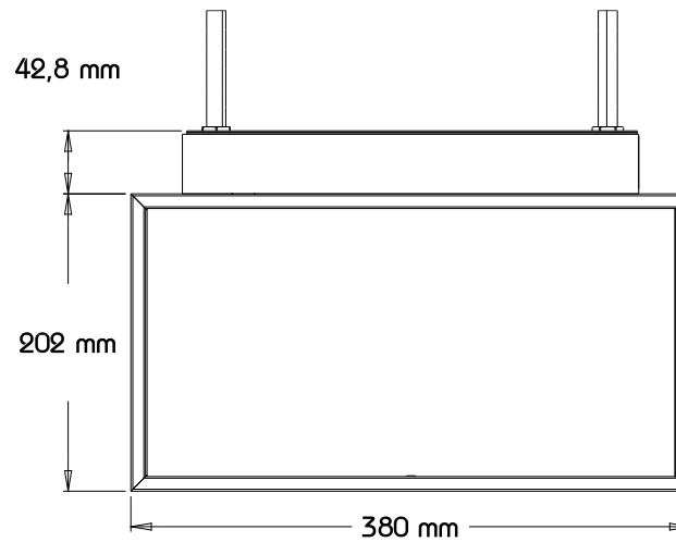
Ansicht Hinten
