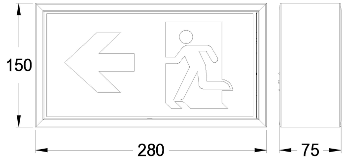
Maßzeichnung (Angaben in mm)
