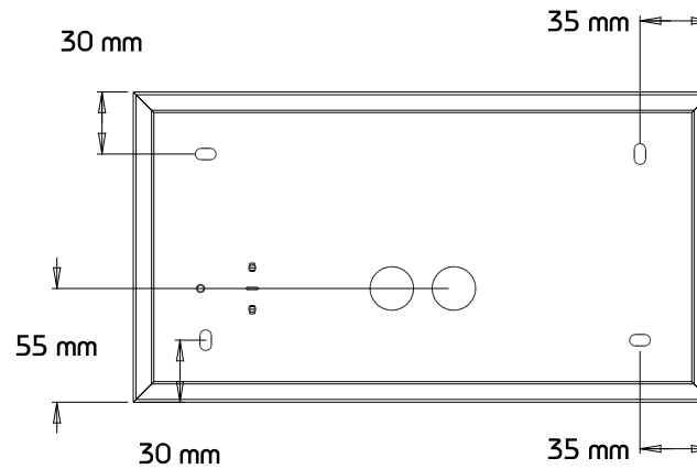
Ansicht Hinten
