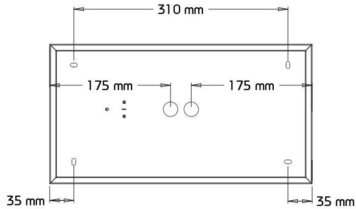
Ansicht Hinten
