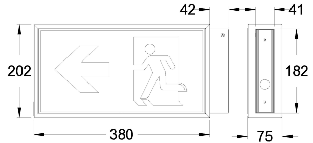
Maßzeichnung (Angaben in mm)
