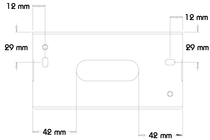
Ansicht Hinten
