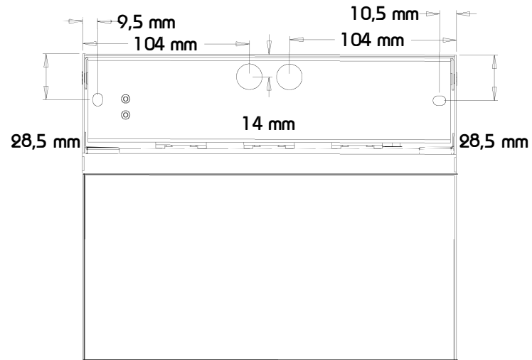
Ansicht Hinten
