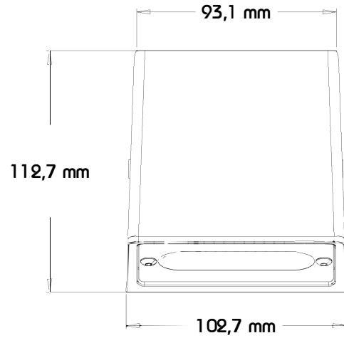
Ansicht Vorne
