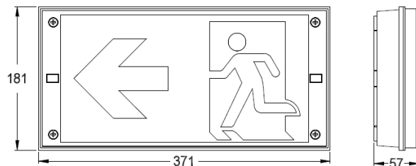
Maßzeichnung (Angaben in mm)
