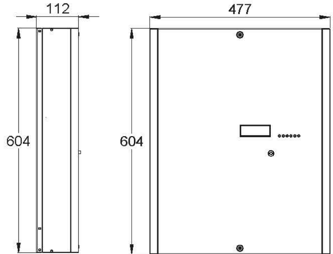
Maßzeichnung (Angaben in mm)
